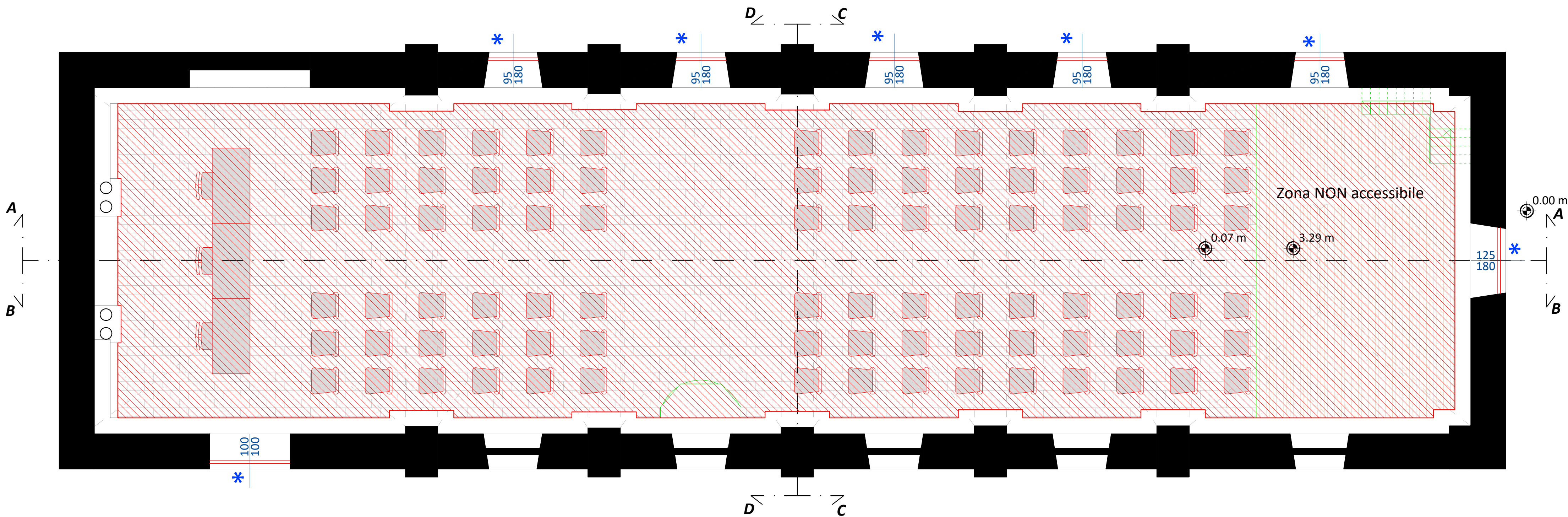
PIANTA QUOTA +5.80 m - COSTRUZIONI
